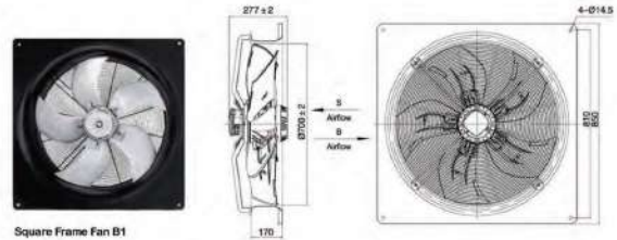
Square Frame Fan B1
